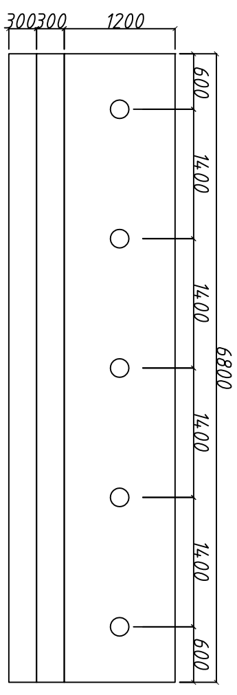
旗台俯视图
