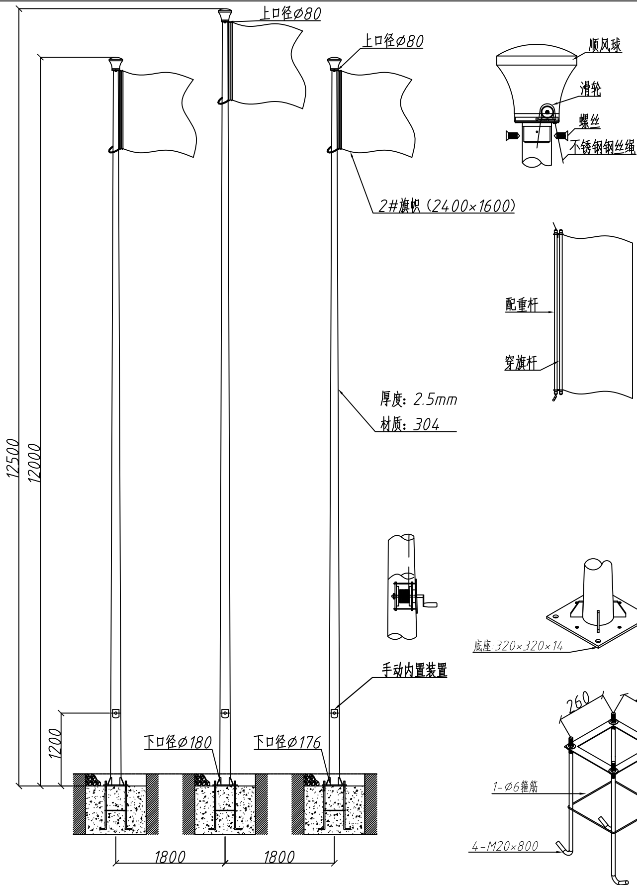
12.5米12米手动内 置锥形旗杆图
